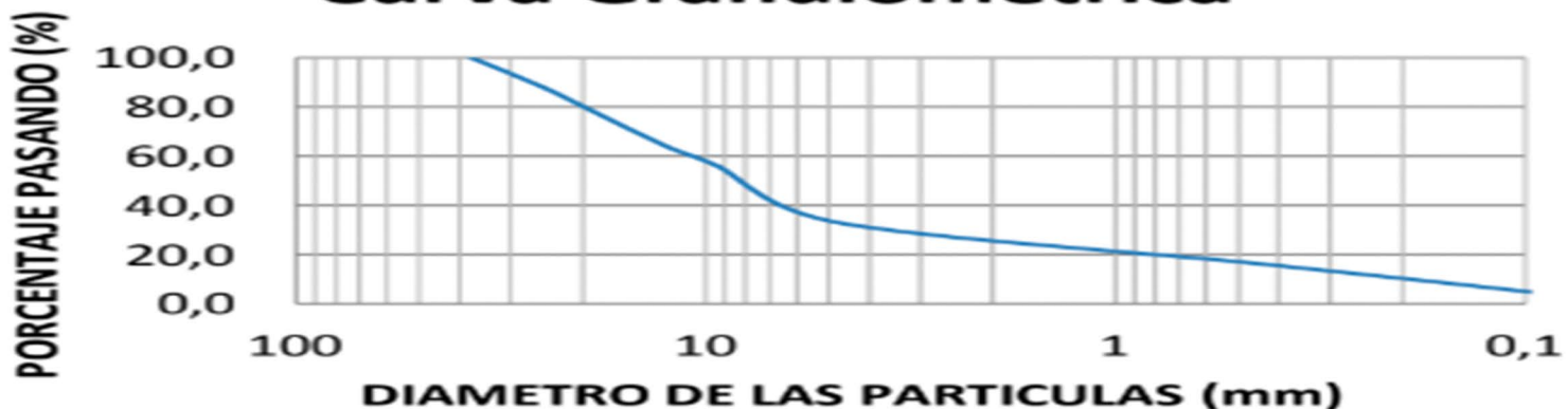
Curva Granulométrica
