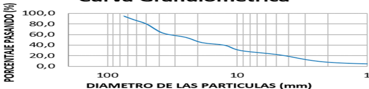
Curva Granulométrica
